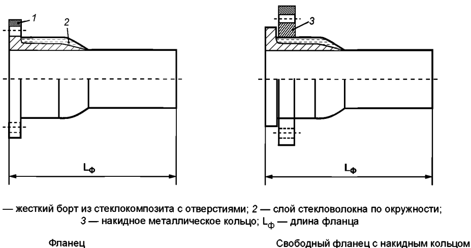
Рисунок 8 — Фланцы
